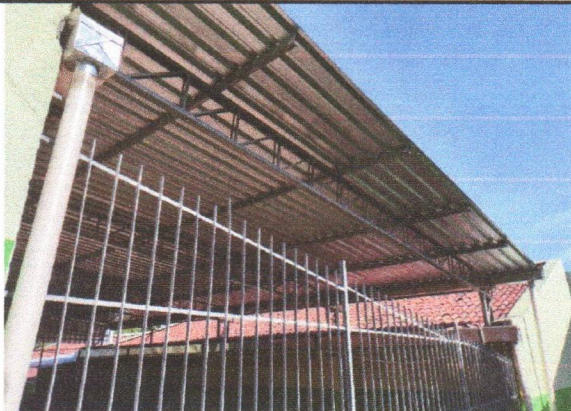
ESCOLA MUNICIPAL APOLÔNIO SALES - INSTALAÇÃO DE ESTRUTURA METÁLICA PARA COBERTA
