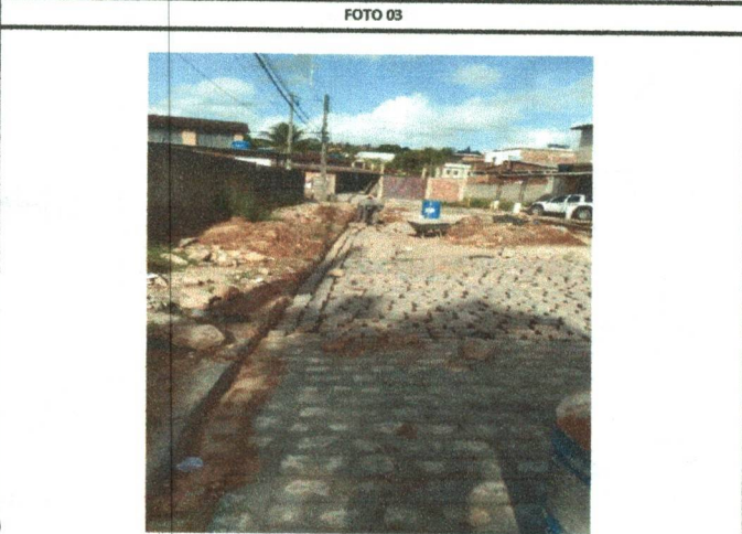
REASSENTAMENTO DE PARALELEPÍPEDOS, REJUNTAMENTO COM ARGAMASSA, COM REAPROVEITAMENTO DOS PARALELEPÍPEDOS. AF_12/2020
