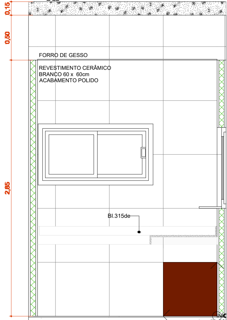
A.M.07 VISTA 1 Escala: 1:25
