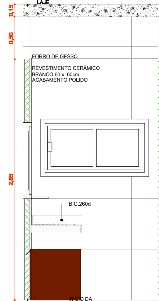
A.M.06 VISTA 3 Escala: 1:25
