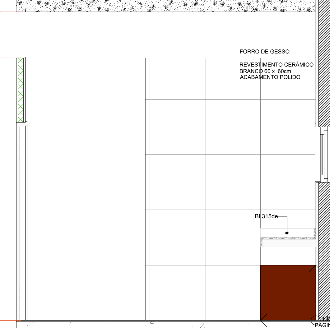
A.M.07 VISTA 2 Escala: 1:25
