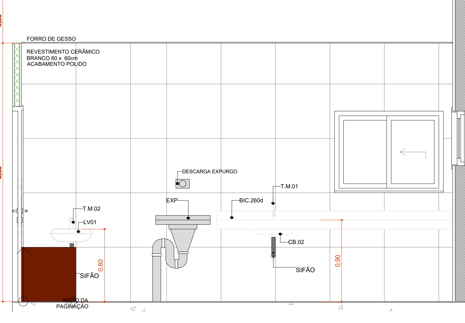
A.M.06 VISTA 2 Escala: 1:25
