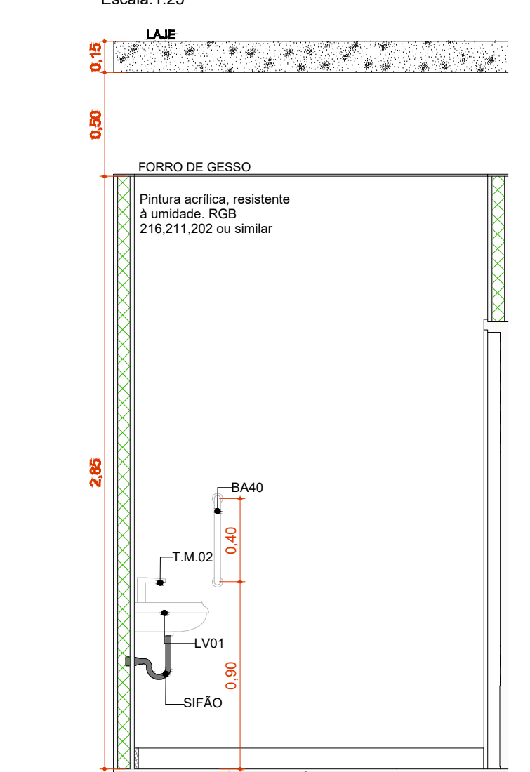
A.M.05 VISTA 4 Escala: 1:25
