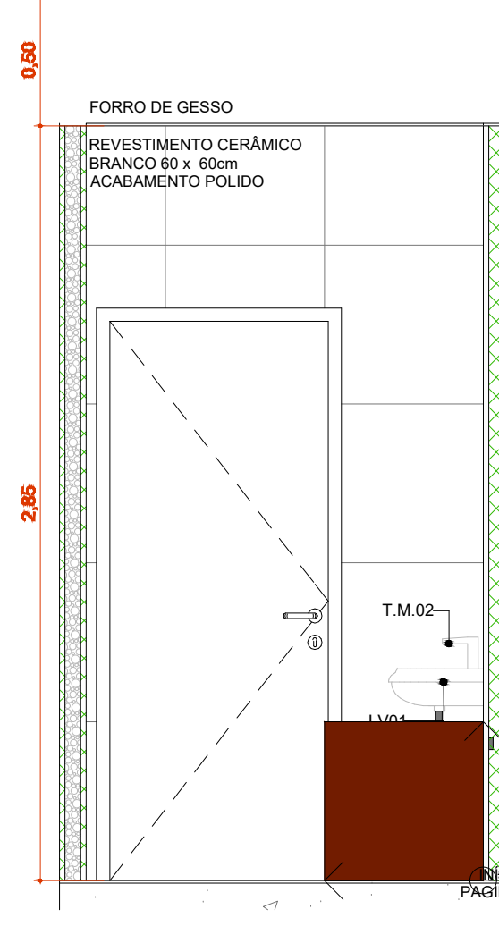
A.M.06 VISTA 1 Escala: 1:25
