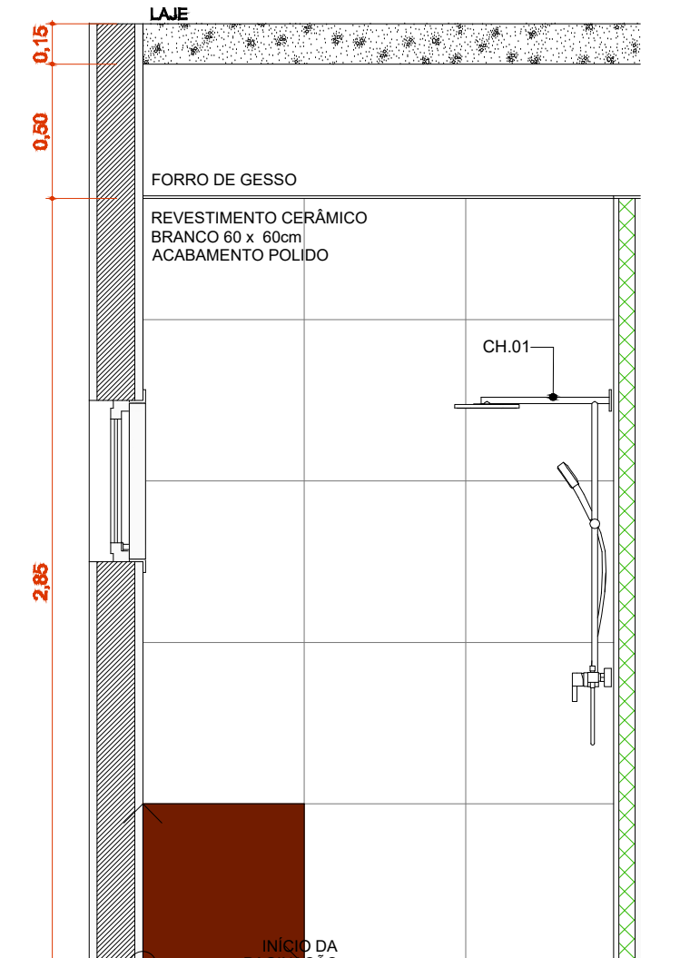
A.M.08 VISTA 1 Escala: 1:25
