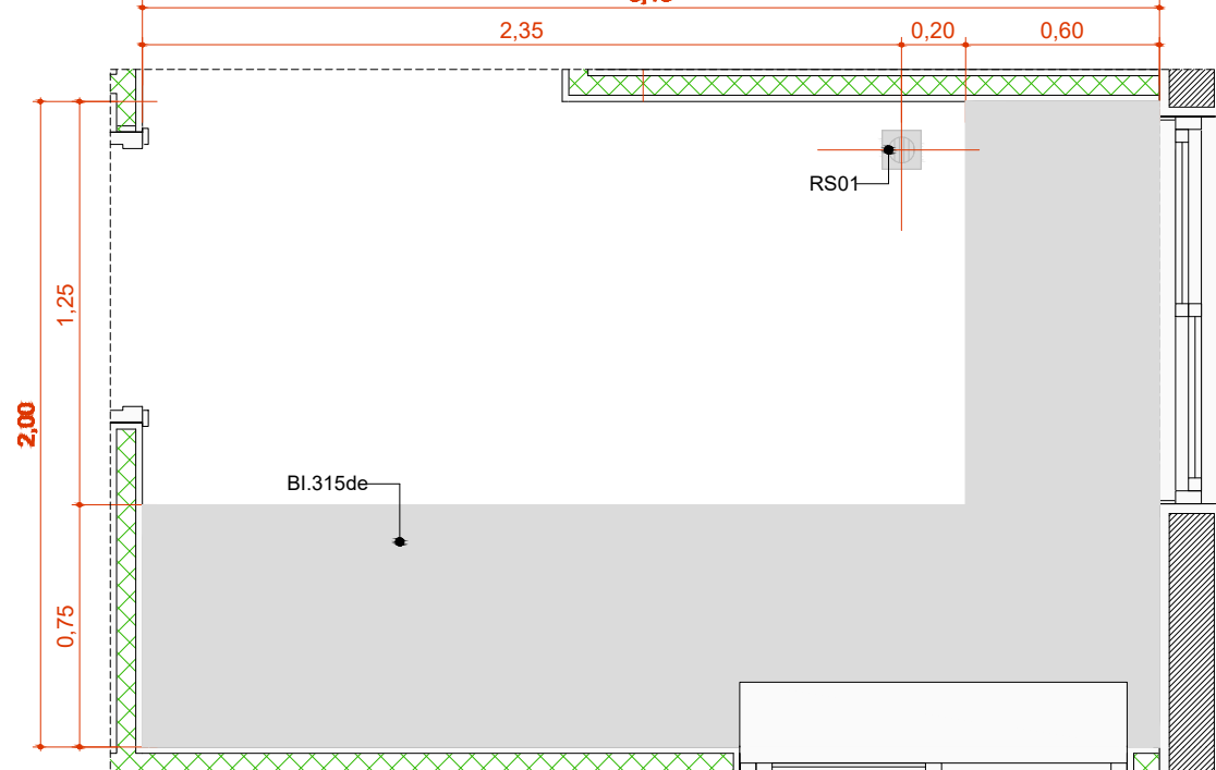
A.M.07 Esterilização Escala: 1:25
