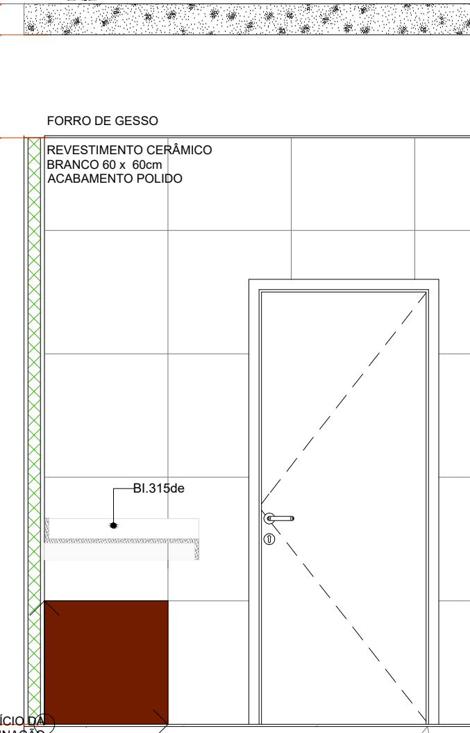
A.M.07 VISTA 4 Escala: 1:25
