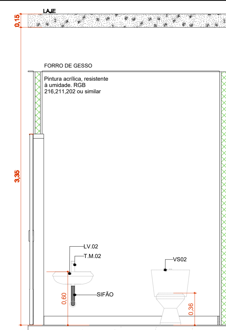
A.M.01 VISTA 4 Escala: 1:25
