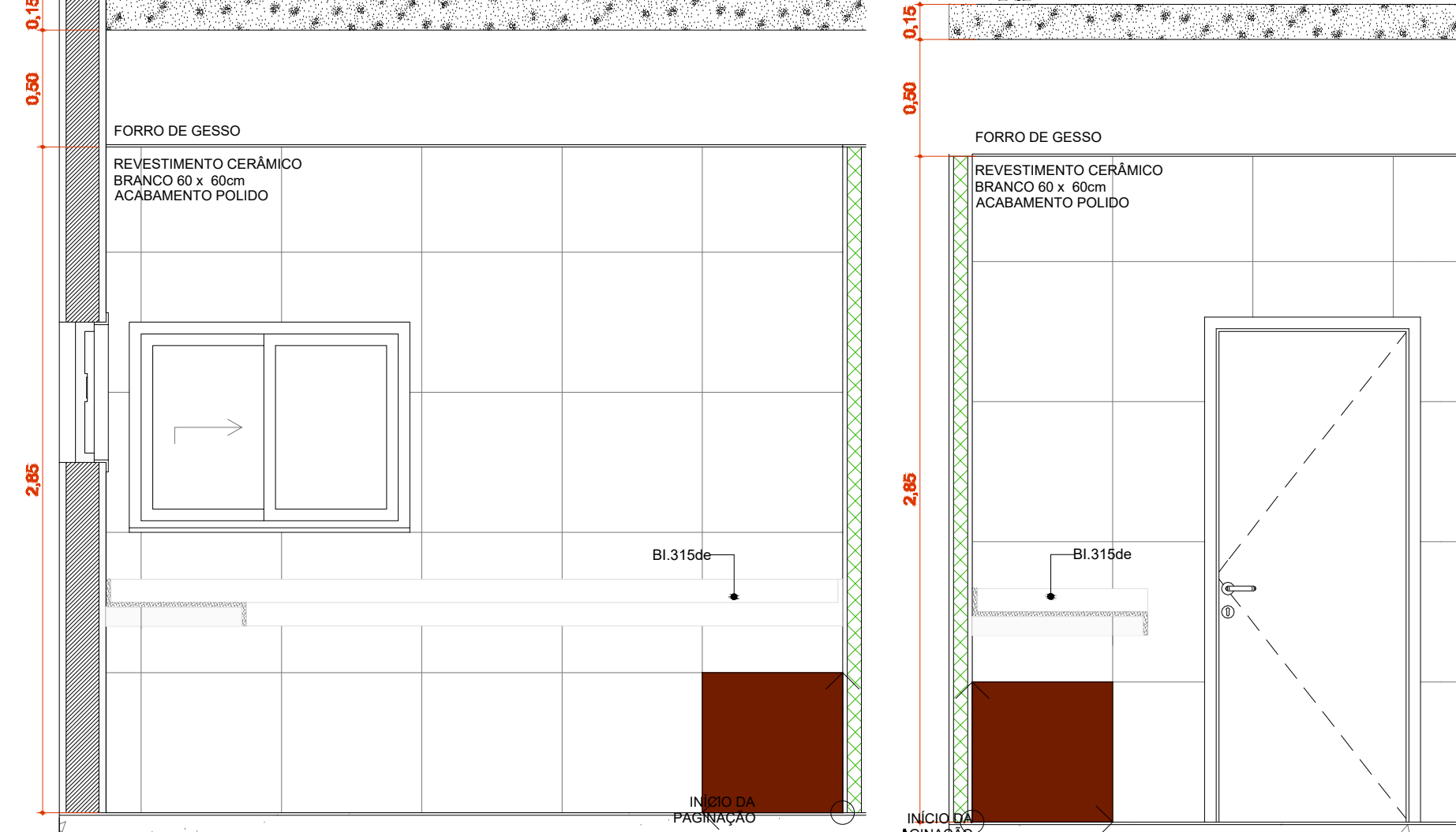
A.M.07 VISTA 3 Escala: 1:25
