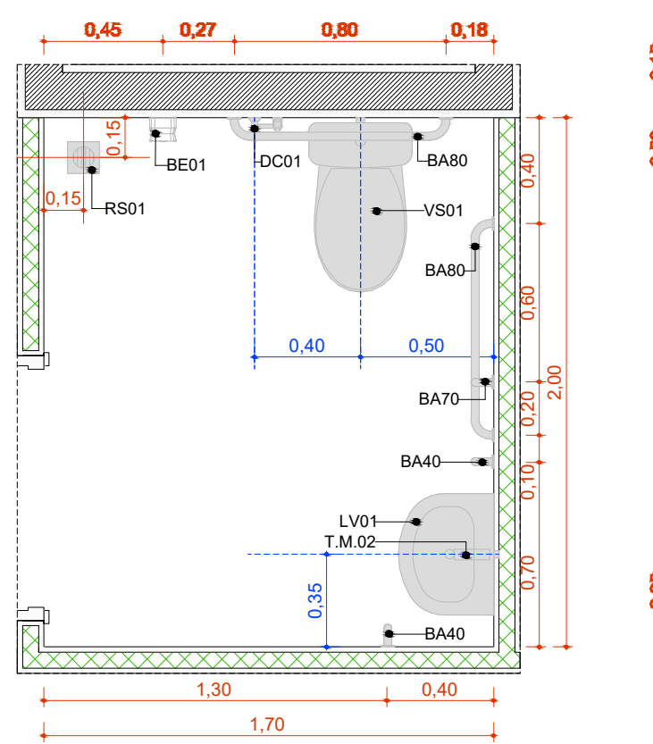
A.M.05 Sanit. PCD Coleta Escala: 1:25
