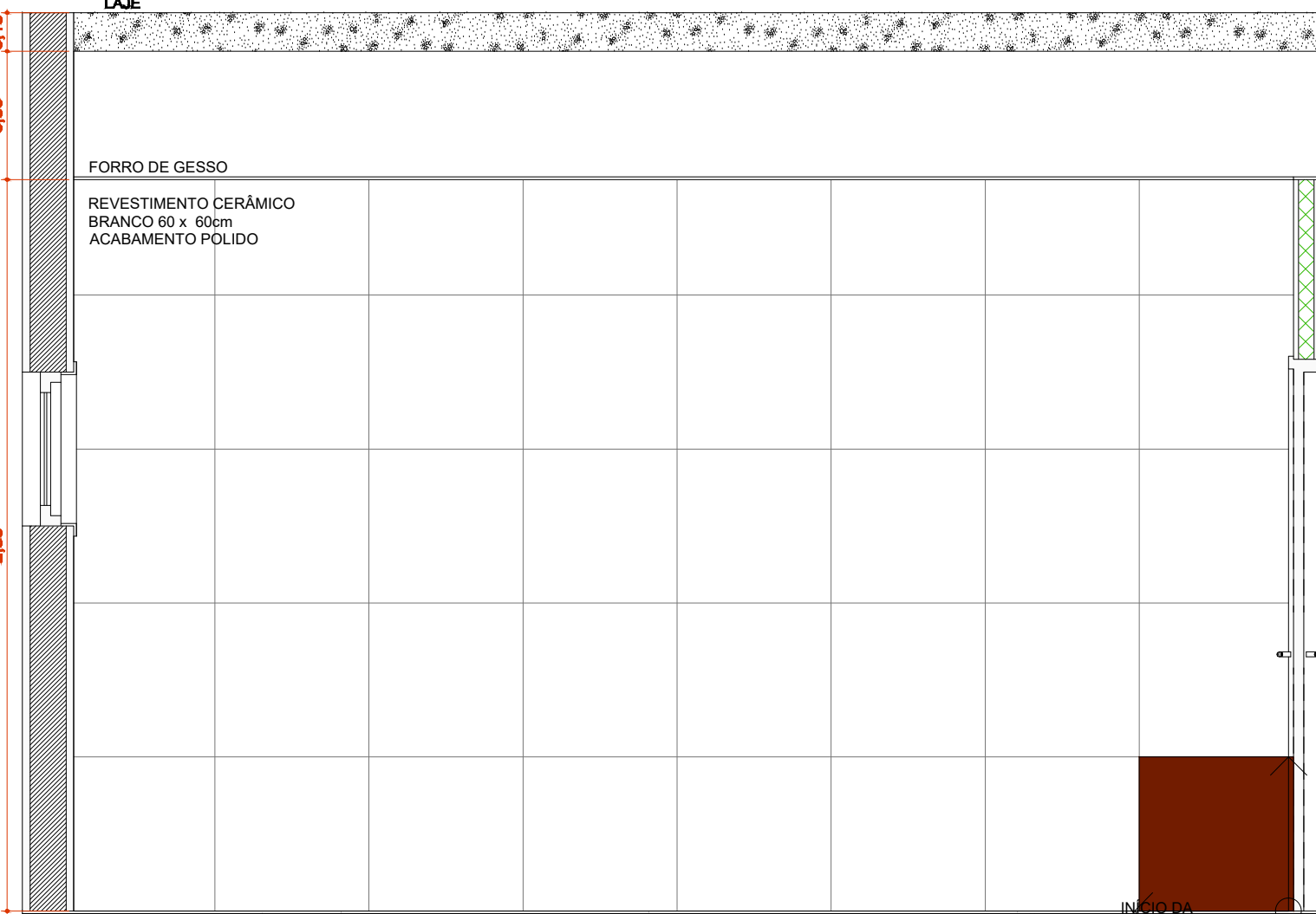
A.M.06 VISTA 4 Escala: 1:25
