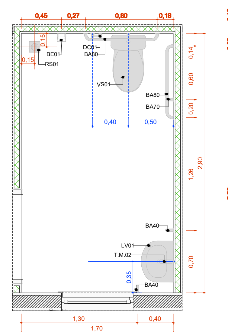
A.M.04 Sanit. PCD Cons. Diferenciado Escala: 1:25
