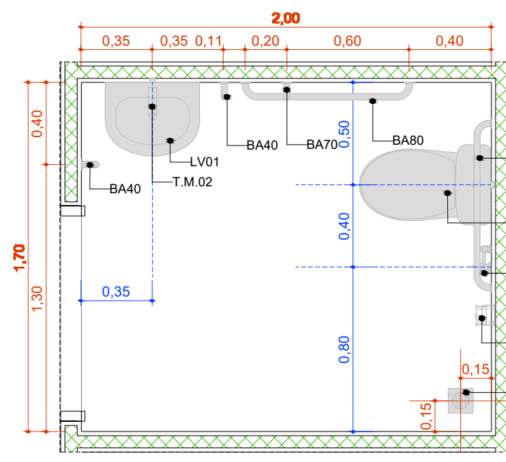
A.M.03 Sanitário PCD Masc. Escala: 1:25
