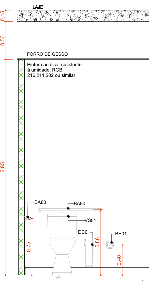
A.M.03 VISTA 1 Escala: 1:25
