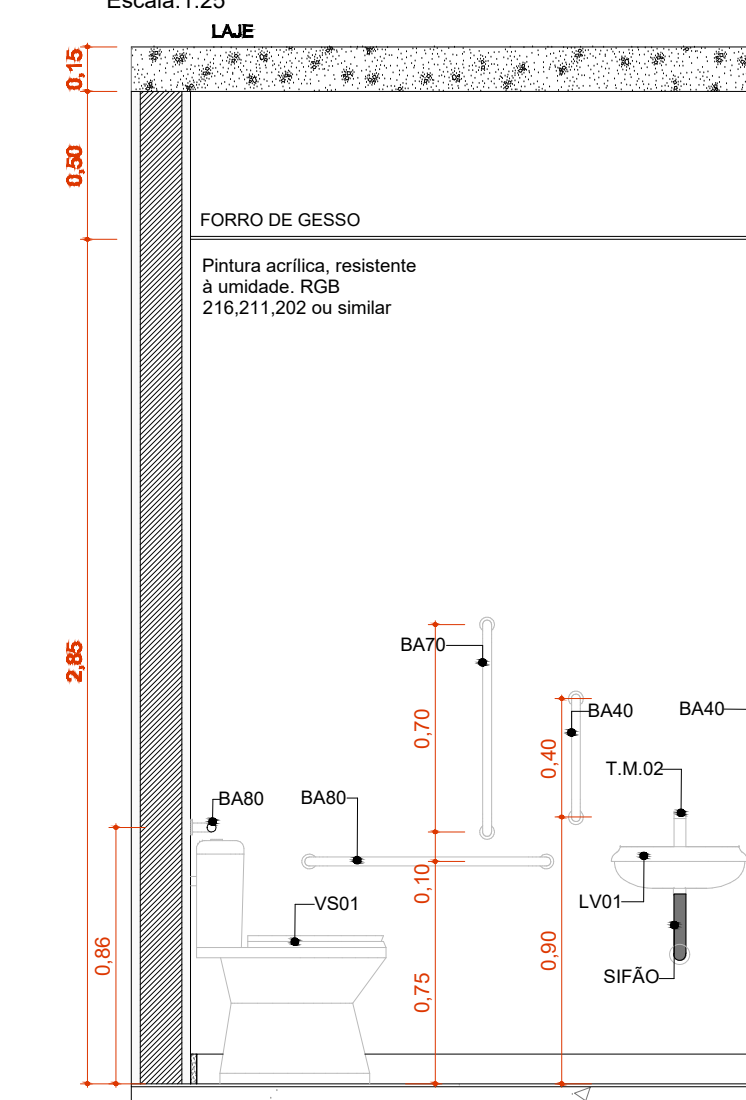
A.M.05 VISTA 3 Escala: 1:25
