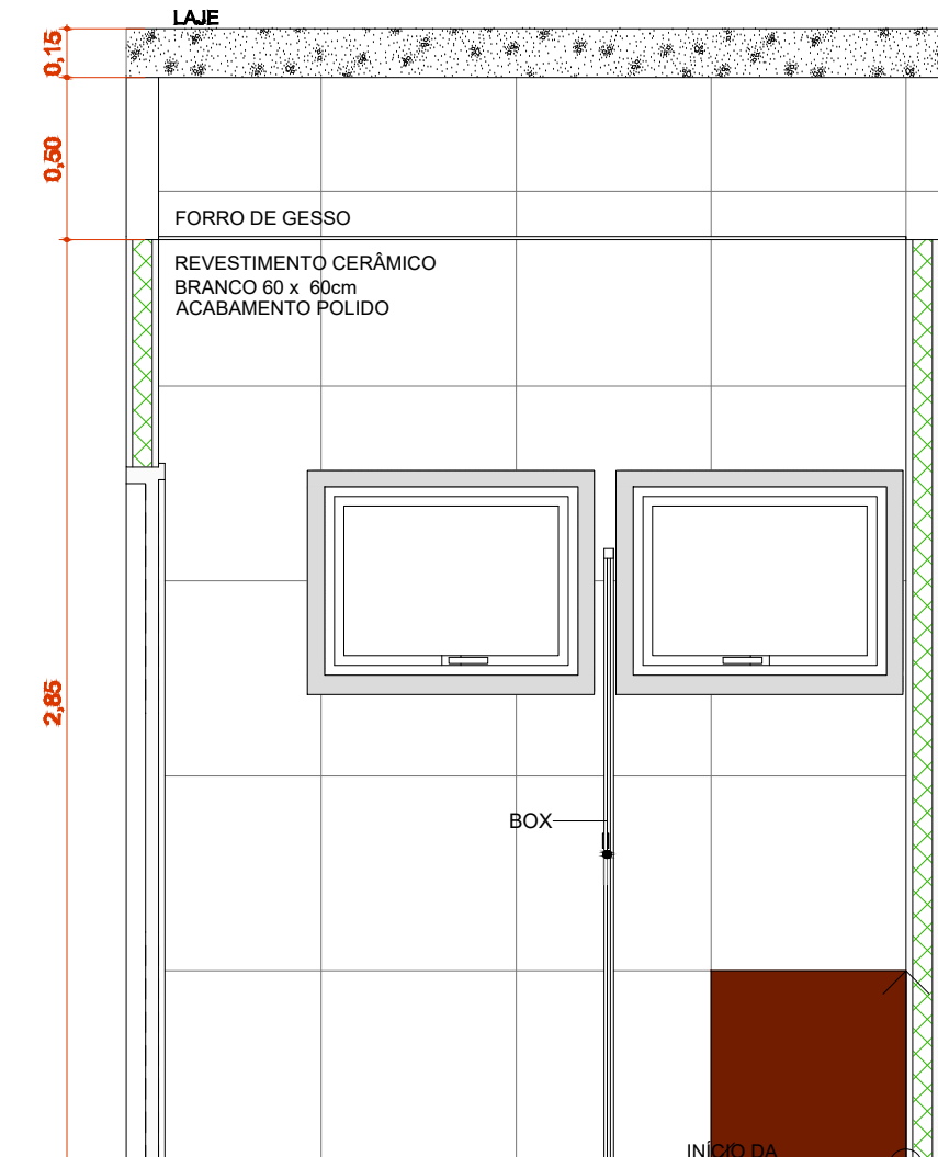
A.M.08 VISTA 2 Escala: 1:25
