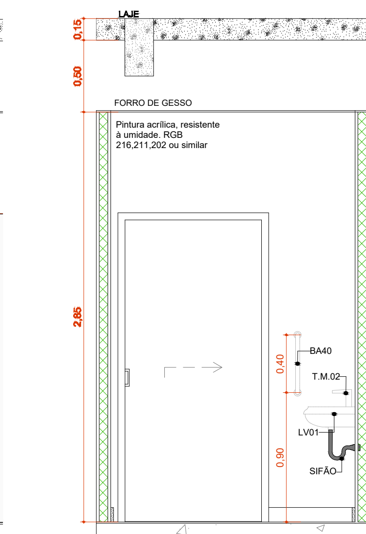
A.M.03 VISTA 4 Escala: 1:25
