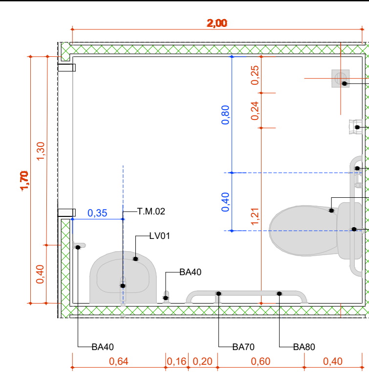
A.M.02 Sanitário PCD Fem. Escala: 1:25
