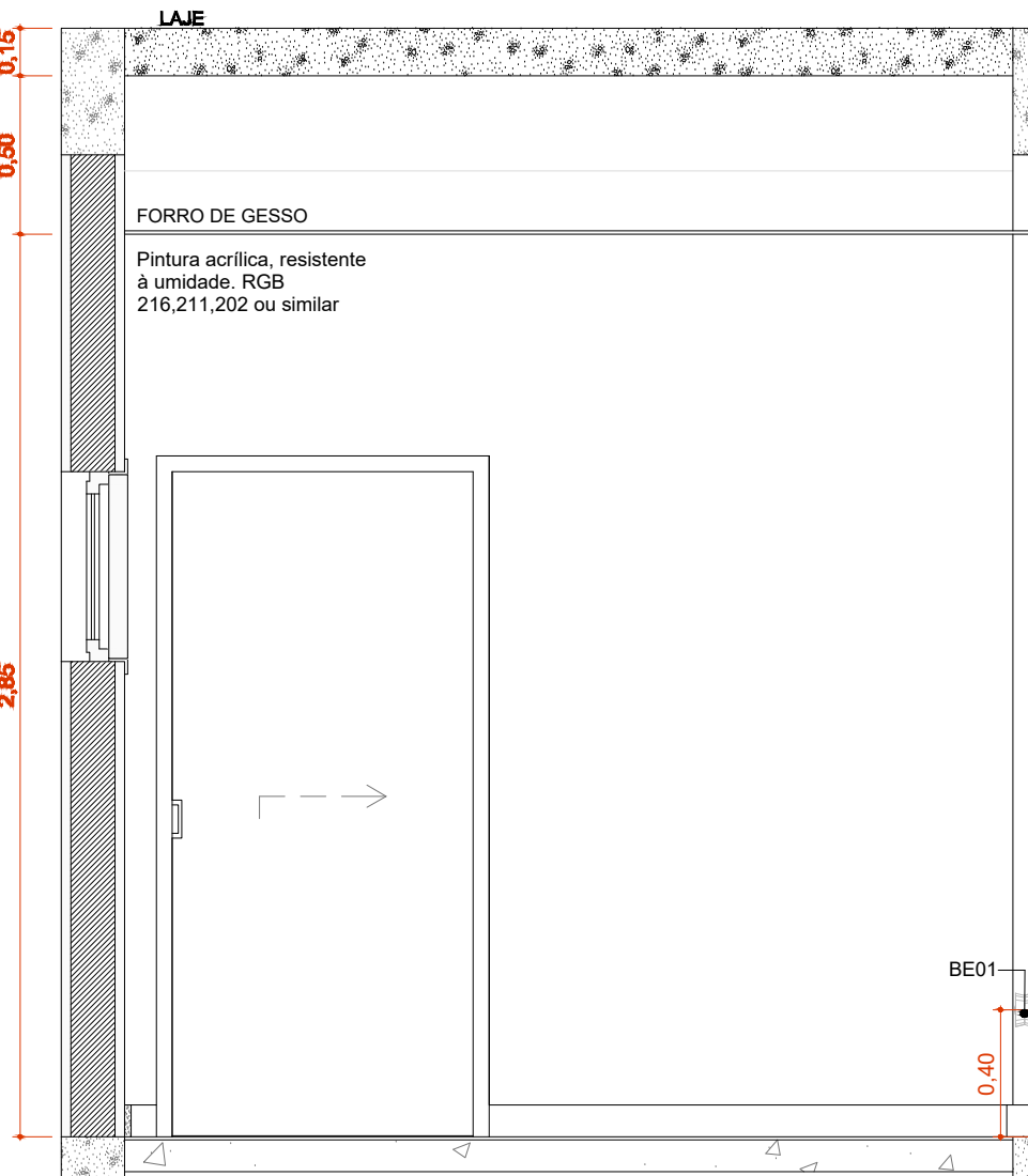
A.M.04 VISTA 1 Escala: 1:25
