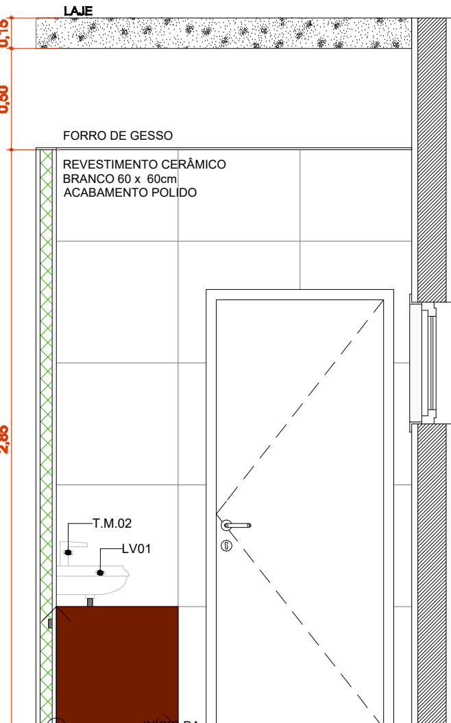
A.M.08 VISTA 4 Escala: 1:25
