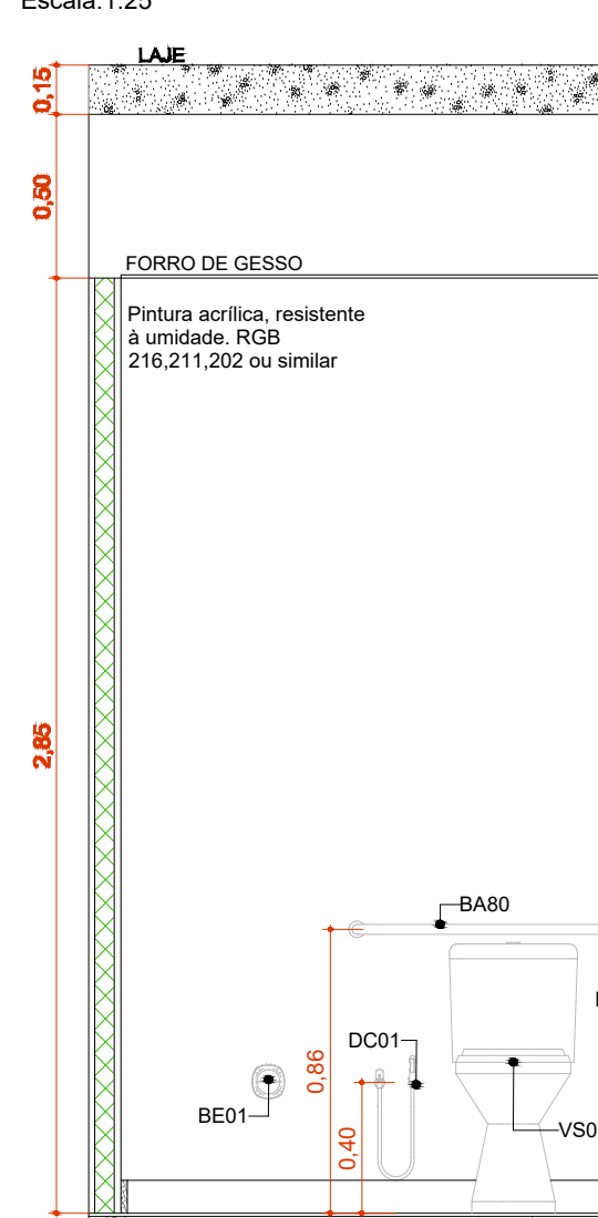
A.M.05 VISTA 2 Escala: 1:25
