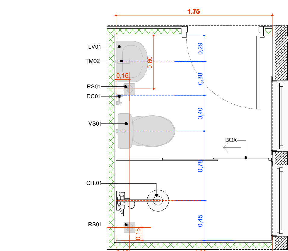
A.M.08 Banh. Func. Masc. Escala: 1:25
