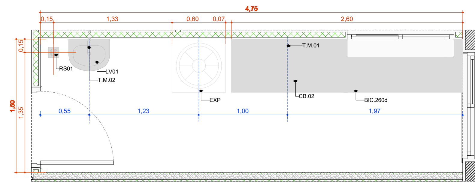
A.M.06 Expurgo Escala: 1:25
