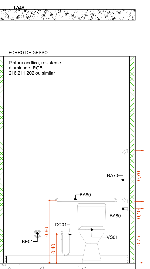
A.M.04 VISTA 2 Escala: 1:25
