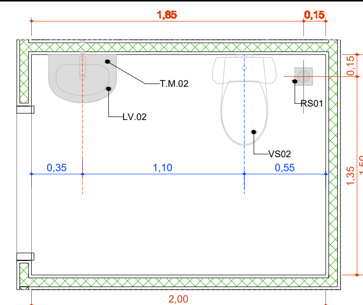
A.M.01 Sanit. Infantil/Faldário Escala: 1:25
