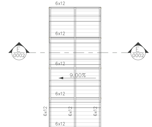
PLANTA DE COBERTURA - NÍVEL 3,65m - 559 LA.1 : 75 V.A.
