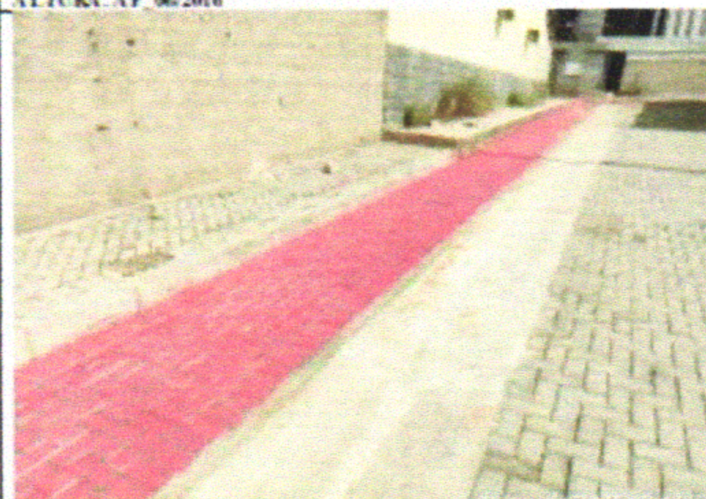
FOTO 15 - SARJETÃO DR 8, DE CONCRETO USINADO, MOLDADA IN LOCO EM TRECHO RETO, 90 CM BASE X 15 CM ALTURA - CONFORME O PROJETO.
