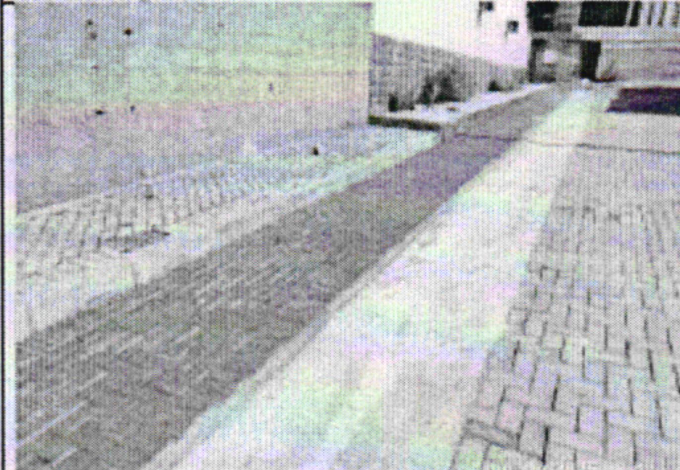
FOTO 15 - SARJETAO DE 8, DE CONCRETO USINADO, MOLDADA IN LOCO EM TRECHO RETO, 90 CM BASE X 15 CM ALTURA - CONFORME O PROJETO.
