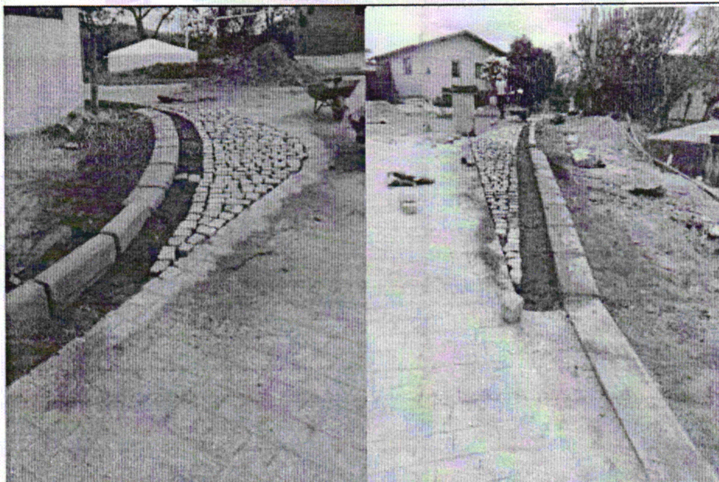
FOTO - 13: EXECUÇÃO DE PAVIMENTAÇÃO
