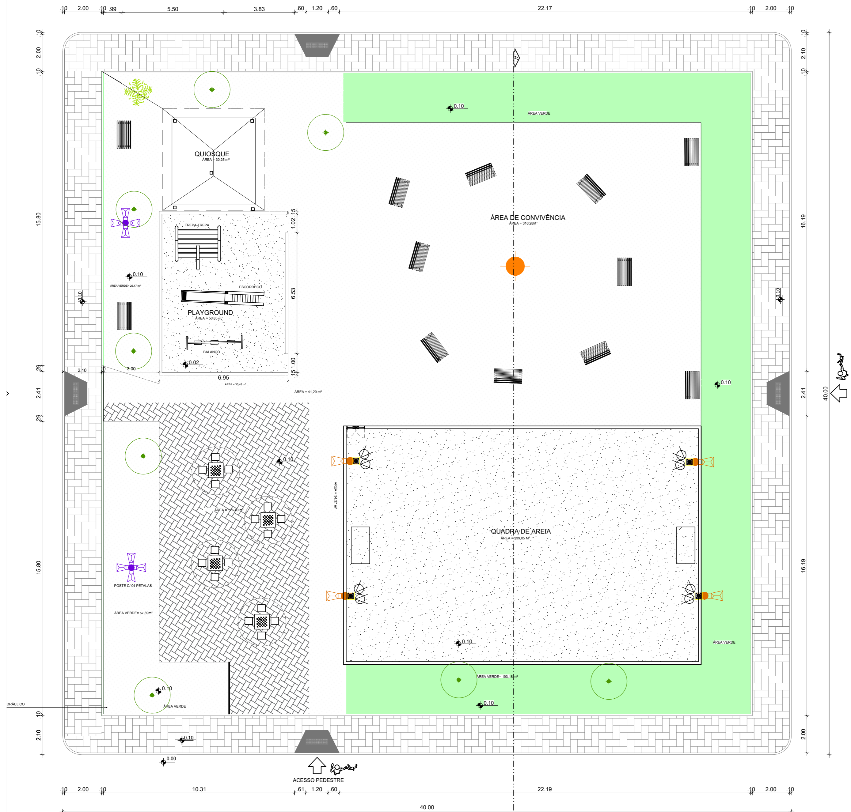
Planta Levantamento Escala: 1:125 Praça Francisca de Paula
