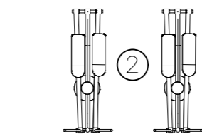
2 PLANTA BAIXA - ESQUI EQUIPAMENTO EM TUBO METÁLICO GALVANIZADO ESCALA: 1/100
