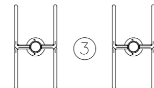
3 PLANTA BAIXA - SIMULADOR DE ESCADA EQUIPAMENTO EM TUBO METÁLICO GALVANIZADO ESCALA: 1/100
