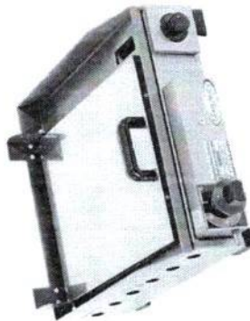
Chapa Extra Prática 40x40 Com Prensa e Com Gaveta 1 Queimador Altura: 15,5 cm Profundidade: 49,0 cm Frente: 40,0 cm Código: 11029 / 11008
