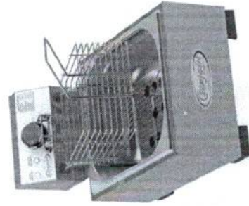
Fritador 5 Litros Elétrico Acompanha Cesto Altura: 34,5 cm Profundidade: 52,0 cm Frente: 28,0 cm Código: 10013
