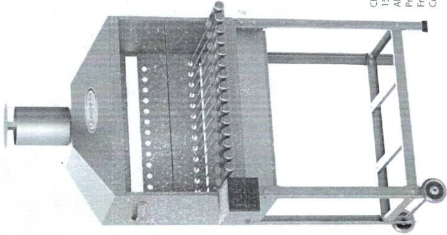
Churrasqueira Brava 15 Espetos Altura: 161,5 cm Profundidade: 57,0 cm Frente: 72,0 cm Código: 9372
