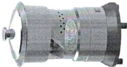
Extrator Plus Total Alumínio 1/4 Cv Altura: 34,0 cm Diâmetro: 19,0 cm Código: 70004-1
