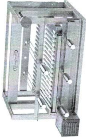
Elevante 5 Espetos com motor Altura: 43,5 cm Profundidade: 50,0 cm Frente: 71,5 cm Código: 9431
