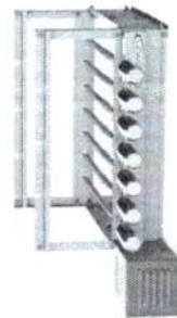
Itagrill Dupla Linear 7 Espetos * Espetos Espadas Altura: 28,5 cm Frente: 48,5 cm Frente com Motor: 58,5 cm Código: 9326
