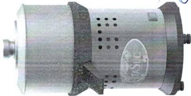
Extrator Plus Inox Caçamba Inox Bica Plástica 1/4 Cv Altura: 29,0 cm Diâmetro: 19,0 cm Código: 70004-5
