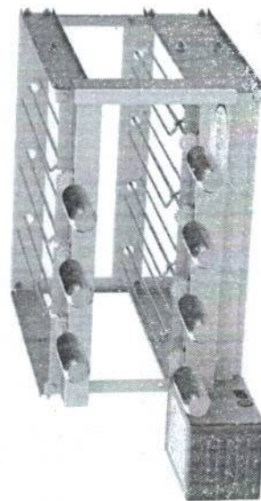
Itagrill Dupla 9 Espetos Altura: 31,0 cm Profundidade: 65,0 cm Frente: 60,0 cm Frente com Motor: 70,0 cm Código: 9213
