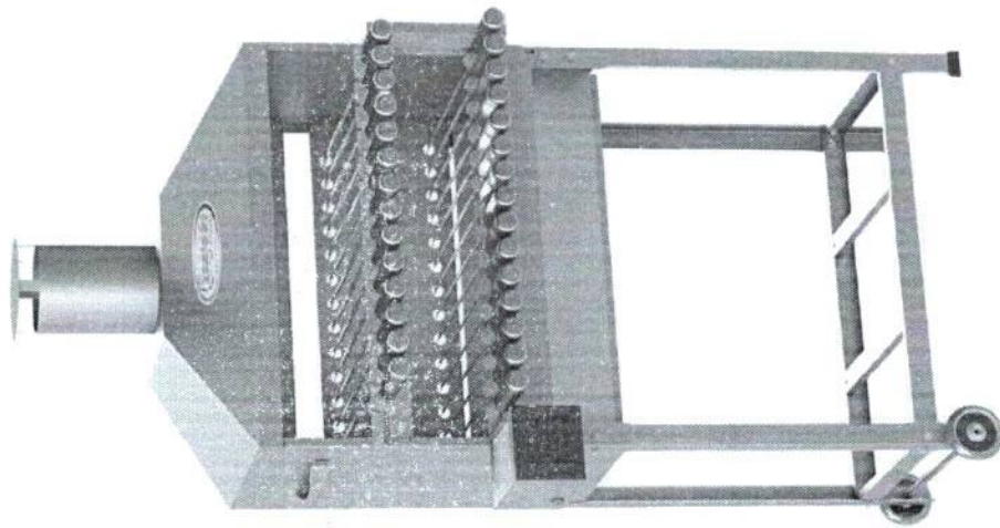
Churrasqueira Brava Dupla 29 Espetos Altura: 161,5 cm Profundidade: 57,0 cm Frente: 83,0 cm Código: 9373
