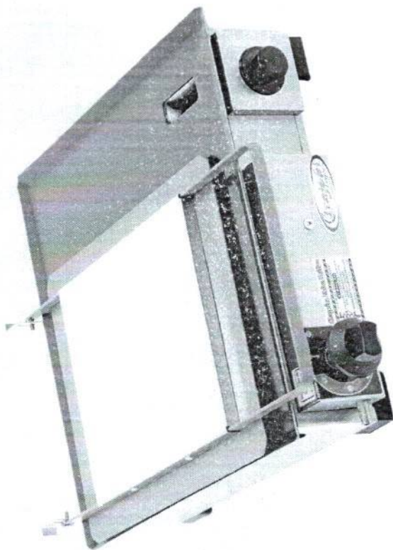
Sanduicheira 430x430 Com Prensa e Com Gaveta 1 Queimador Altura: 15,0 cm Profundidade: 49,5 cm Frente: 43,0 cm Código: 11019
