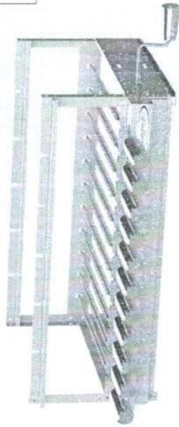
Itagrill Manivela 11 Espetos Altura: 28,5 cm Profundidade: cm Frente: 71,5 cm Frente com Manivela: 93,5 cm Código: 9337
