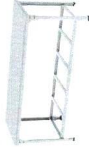
Mesa 1800x700 Tampo Polietileno Estrutura Pintada Altura: 81,0 cm Profundidade: 70,0 cm Frente: 180,0 cm Código: 12028
