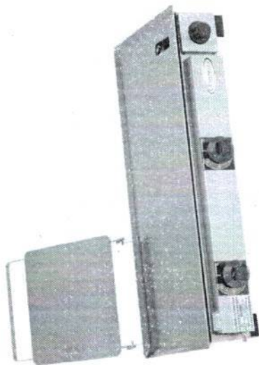
Sanduicheira 700x300 Com Prensa e Com Gaveta 2 Queimadores Altura: 15,0 cm Profundidade: 36,5 cm Frente: 70,0 cm Código: 11017
