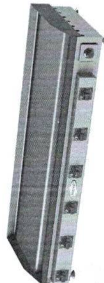
Chapa Profissional 1500x470 6 Queimadores Altura: 22,0 cm Profundidade: 49,0 cm Frente: 150,0 cm Código: 11057
