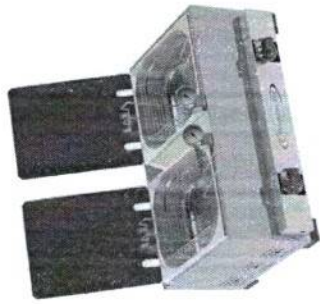
Fritador 10 Litros Gás Acompanha Cesto Altura: 34,5 cm Profundidade: 52,0 cm Frente: 60,0 cm Código: 10031
