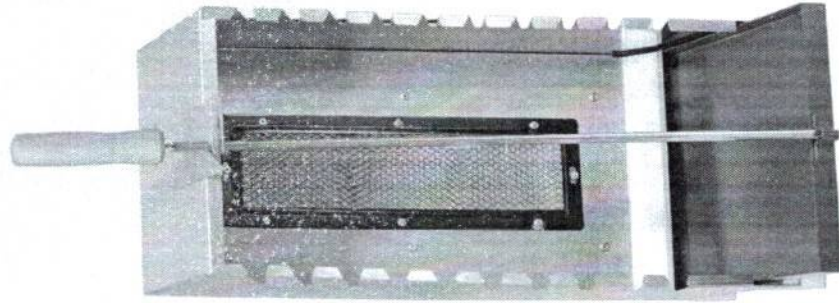
Itagrill Vertical Altura: 63,5 cm Profundidade: 35,5 cm Frente: 20,5 cm Código: 9159
