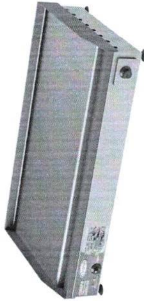
Chapa Profissional 450x470 Altura: 22,0 cm Profundidade: 49,0 cm Frente: 45,0 cm Código: 11044
