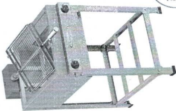
Costeireira Inox C/Infravermelho Medidas Internas Altura: 45,0 cm Profundidade: 63,0 cm Frente: 44,0 cm Medidas Externas Altura: 91,5 cm Profundidade: 99,0 cm Frente: 50,0 cm Código: 9343 / 9366
