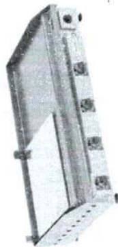
Chapa Profissional 1050x620 Com Prensa - 4 Queimadores Altura: 25,0 cm Profundidade: 64,0 cm Frente: 105,0 cm Código: 11004 / 11028
