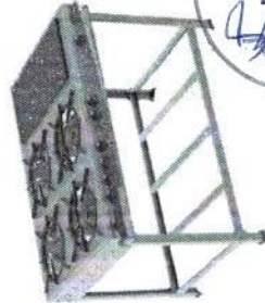
Fogão 4 Bocas Chapa 2 Q. Duplo e 2 Q. Simples Altura: 80,0 cm Profundidade: 83,0 cm Frente: 124,0 cm Código: 4138
