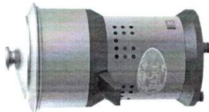
Extrator Plus Inox Caçamba Alumínio Bica Plástica 1/4 Cv Altura: 33,5 cm Diâmetro: 19,0 cm Código: 70004-4
