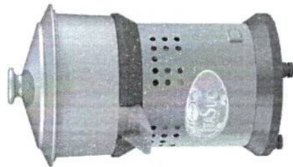
Extrator Plus Inox Caçamba e Bica Alumínio 1/4 Cv Altura: 32,0 cm Diâmetro: 19,0 cm Código: 70004-2
