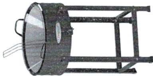
Fritador Grande Pintado Gás Cesto Vendido Separado Altura: 84,5 cm Diâmetro: 45,0 cm Código: 10003 Código Cesto: 137
