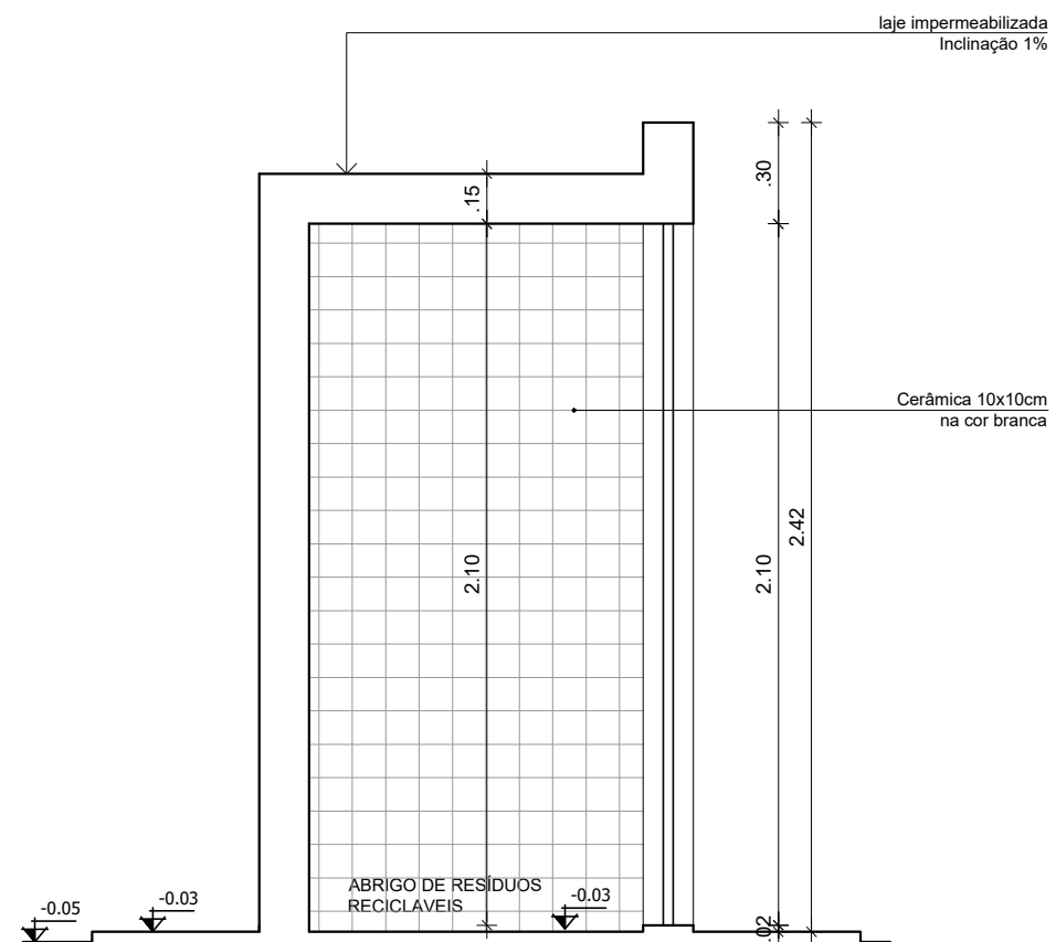
Esc. 1:25 Corte AA Abrigo de resíduos
