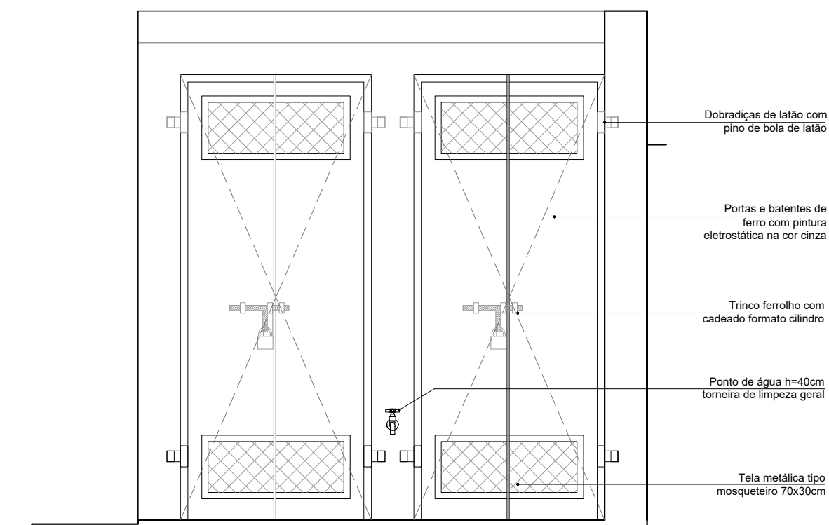
Esc. 1:25 Fachada Abrigo de resíduos
