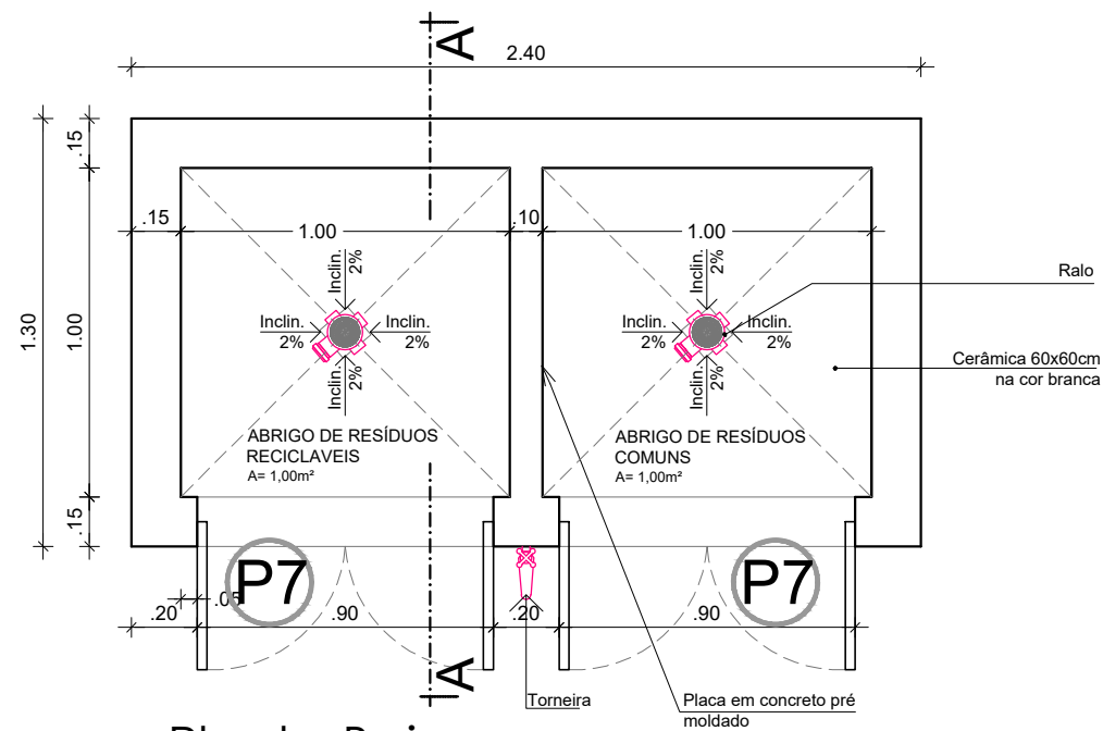
Esc. 1:25 Planta Baixa Abrigo de resíduos
