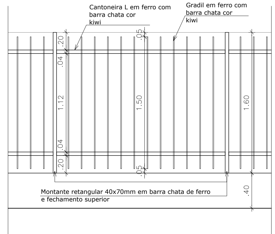
Elevação Esc.1:25 Detalhe Gradil/Muro
