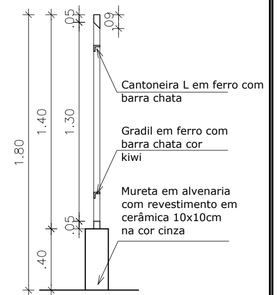
Corte Esc.1:25 Detalhe Gradil/Muro
