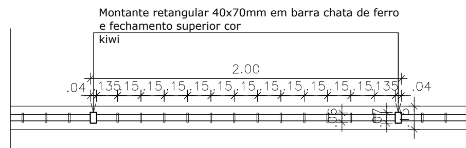
Planta baixa Esc.1:25 Detalhe Gradil/Muro
