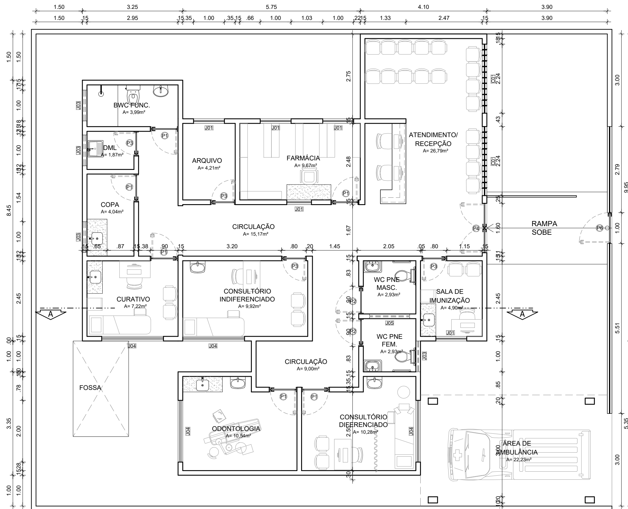
1:75 Planta Baixa E.C. PROPOSTA
