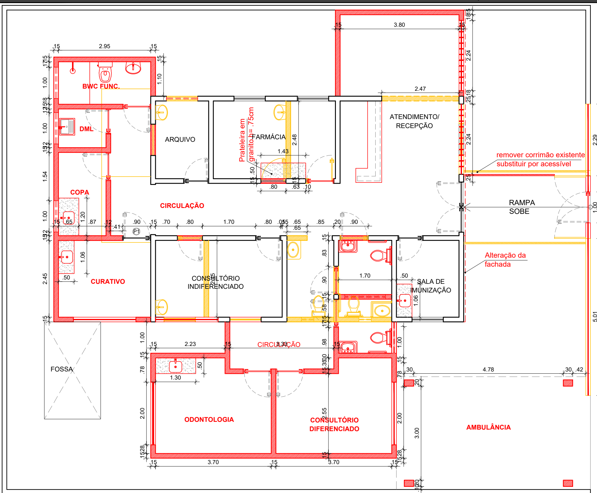
Esc: 1:75 Planta Baixa REFORMA
