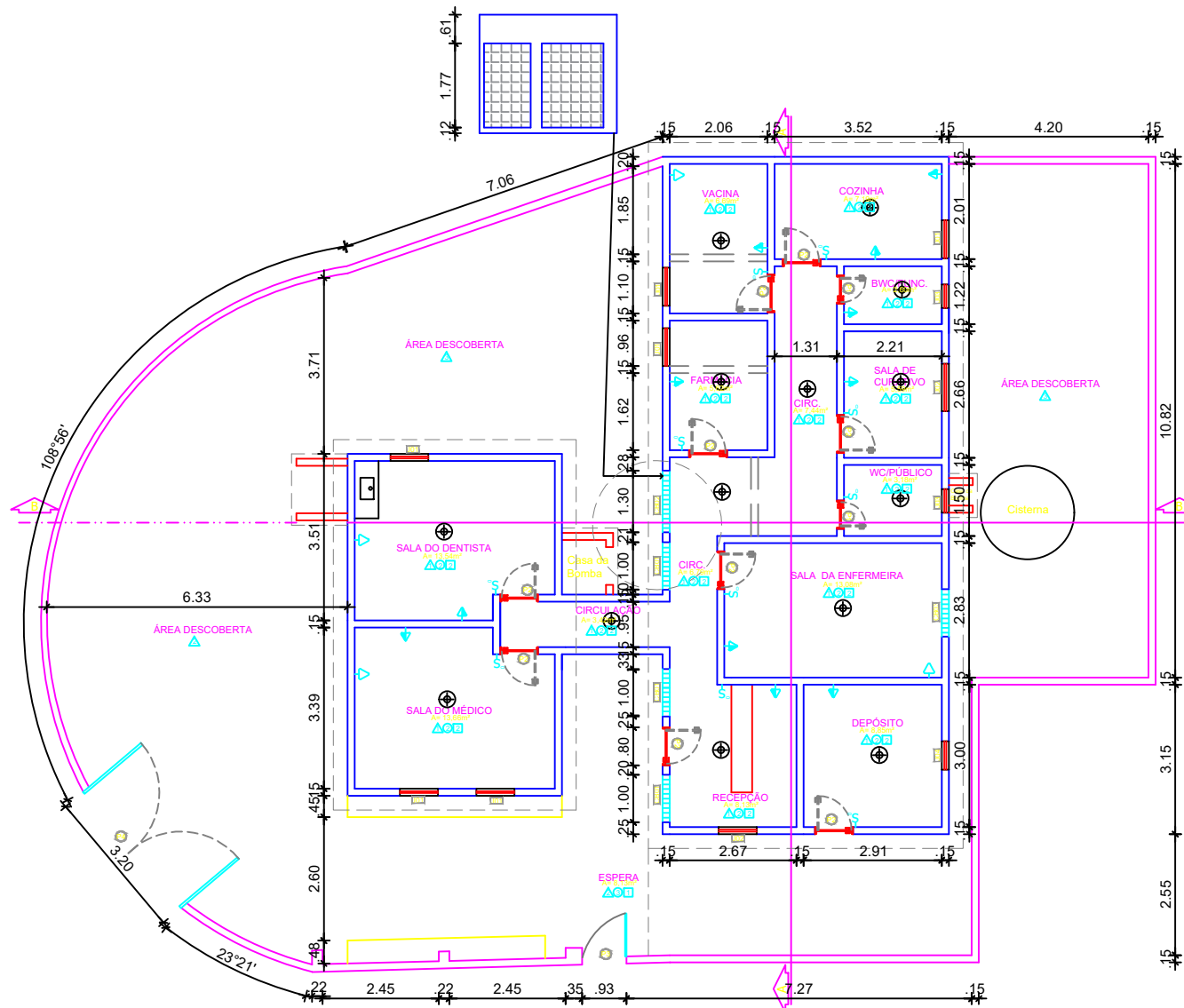
Planta baixa Esc. 1:125 LEVANTAMENTO
